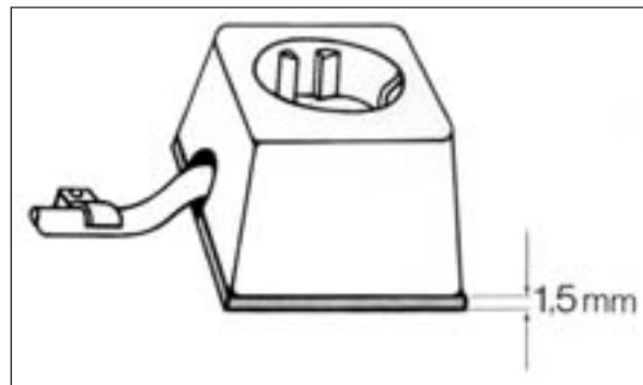
Bild 4: Beispiel für die Anbringung einer Schutzkontakt-Steckdose
