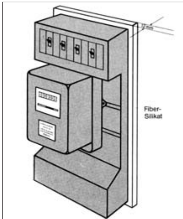
Bild 5: Beispiel für die Anbringung einer Zählertafel
