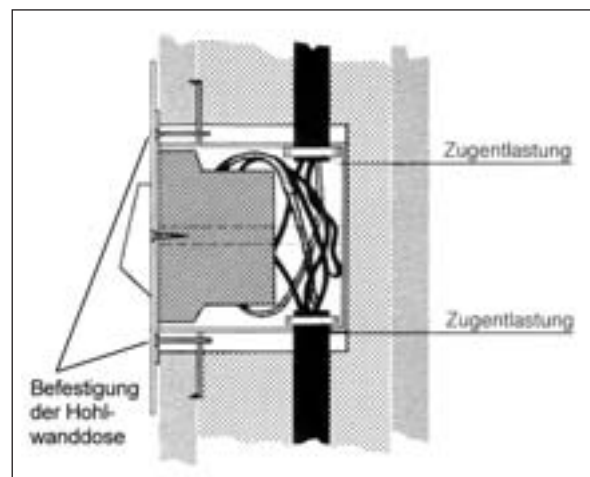
Bild 2: Gerätedose in Hohlwand (Schnitt)
